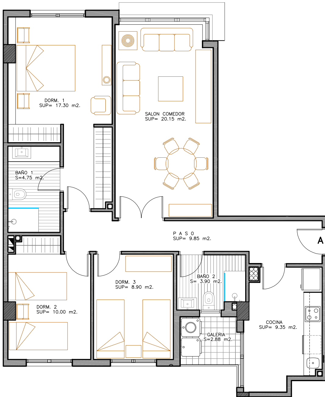
ESCALA 1:75
